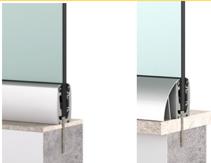
Fijación sobre murete o peto (con o sin anti-escalado)
